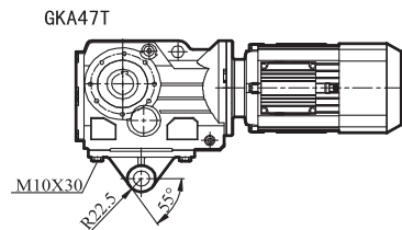
GKA/GKAZ/GKAF47输出轴
