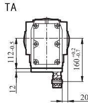
GKH/GKHZ/GLHF47输出轴
