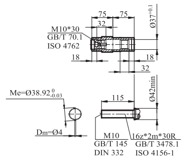
GKV/GKVZ/GKVF47输出轴
