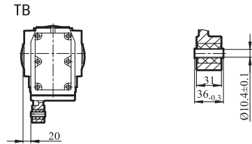
GKV/GKVZ/GKVF47输出轴
