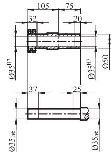
GKH/GKHZ/GLHF47输出轴
